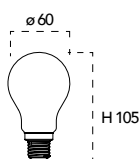
Lampada LED filamento 8W 230V
